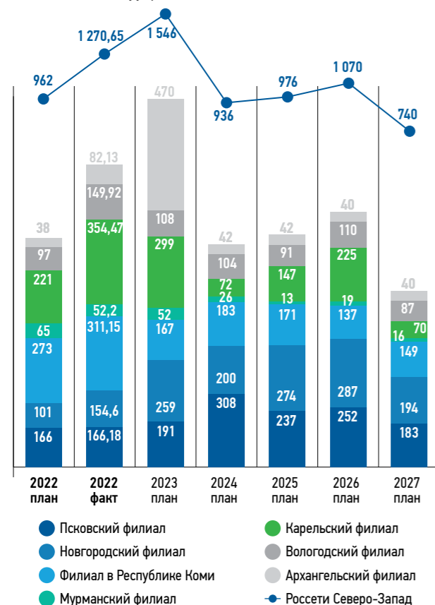
Динамика ввода линий электропередачи на 2022–2027 годы, км
