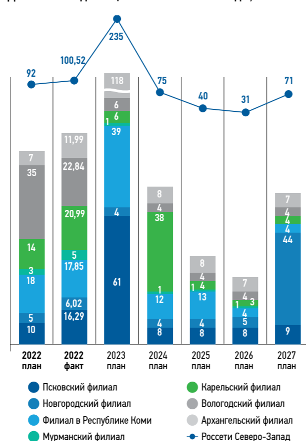
Динамика ввода мощности на 2022–2027 годы, МВА
